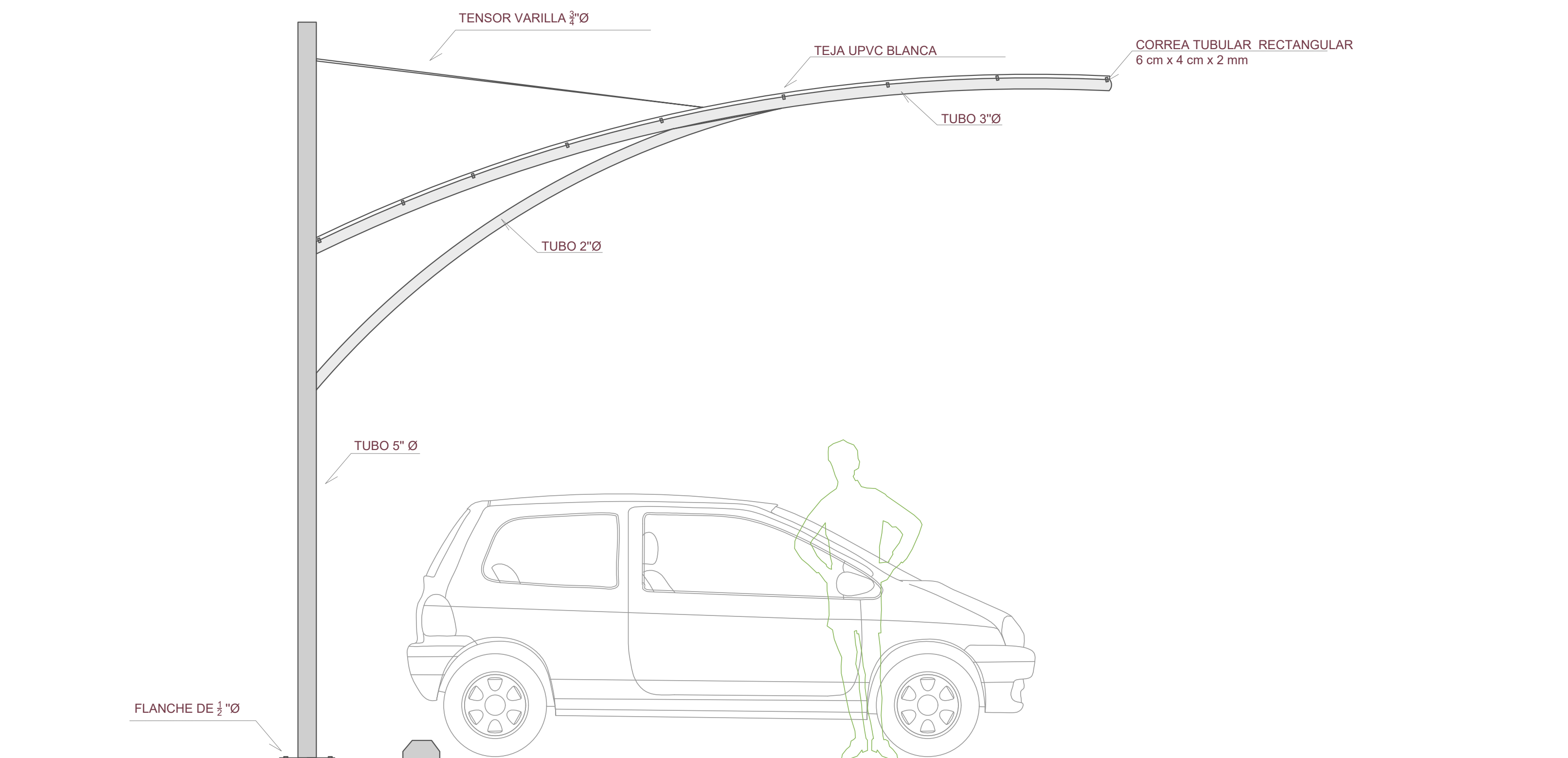
ESTRUCTURA PARQUEADERO ESC : 1: 10
